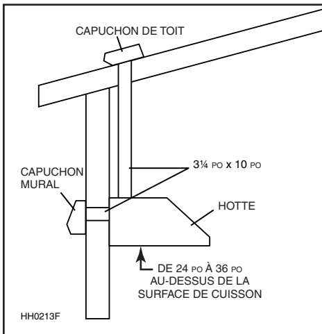
INSTALLATION DE CONDUITS RECTANGULAIRES AVEC VENTILATEUR INTÉRIEUR MODÈLE P5 (SIMPLE)
