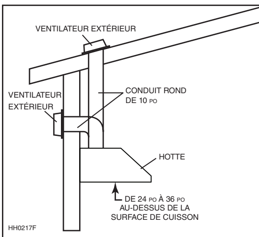
INSTALLATION TYPE AVEC VENTILATEUR EXTÉRIEUR MODÈLE EB9 OU EB15
