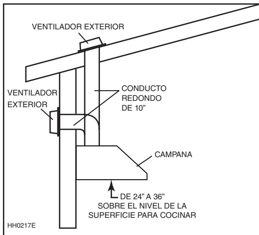
INSTALACIÓN ESTÁNDAR CON VENTILADOR EXTERIOR MODELO EB9 O EB15
