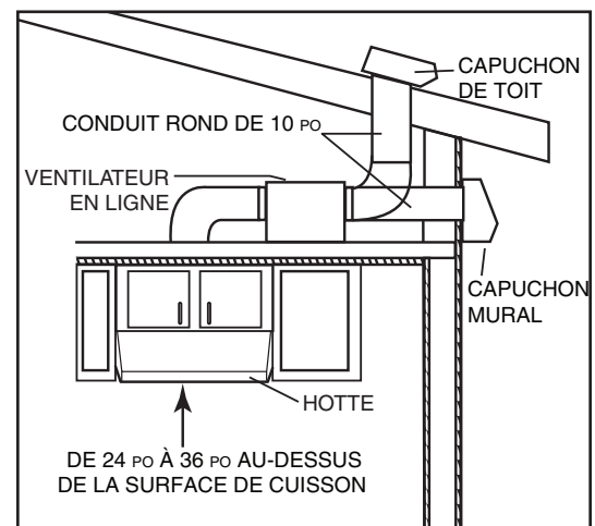
INSTALLATION TYPE AVEC VENTILATEUR EN LIGNE MODÈLE ILB6, ILB9 OU ILB11
