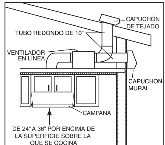
INSTALACIÓN ESTÁNDAR CON VENTILADOR EN LÍNEA MODELO ILB6, ILB9 O ILB11
