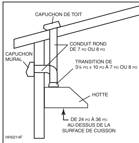
INSTALLATION DE CONDUITS CIRCULAIRES DE 7 PO OU DE 8 PO AVEC VENTILATEUR INTÉRIEUR MODÈLE P5 (SIMPLE)
