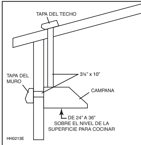
INSTALACIÓN CON CONDUCTO RECTANGULAR CON VENTILADOR INTERIOR MODELO P5 (SIMPLE)
