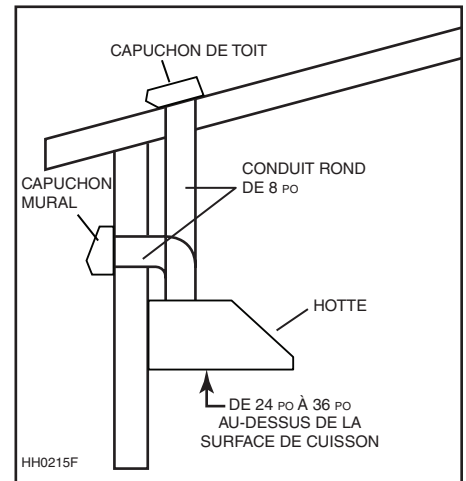
INSTALLATION DE CONDUITS CIRCULAIRES DE 8 PO AVEC VENTILATEUR INTÉRIEUR MODÈLE iQ6
