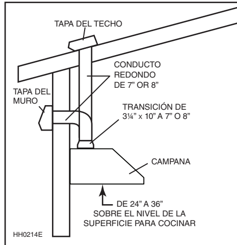
INSTALACIÓN CON CONDUCTO REDONDO DE 7" O 8" CON VENTILADOR INTERIOR MODELO P5 (SIMPLE)
