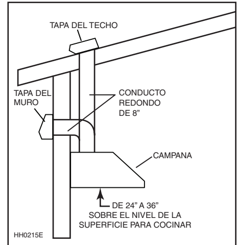
INSTALACIÓN CON CONDUCTO REDONDO DE 8" CON VENTILADOR INTERIOR MODELO iQ6 (SIMPLE)
