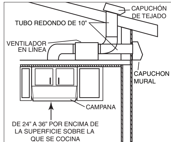
INSTALACIÓN HABITUAL CON EL VENTILADOR EN LÍNEA ILB6, ILB9 O ILB11
