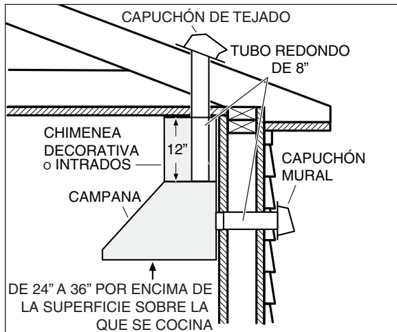
INSTALACIÓN HABITUAL CON EL VENTILADOR SIMPLE iQ6
