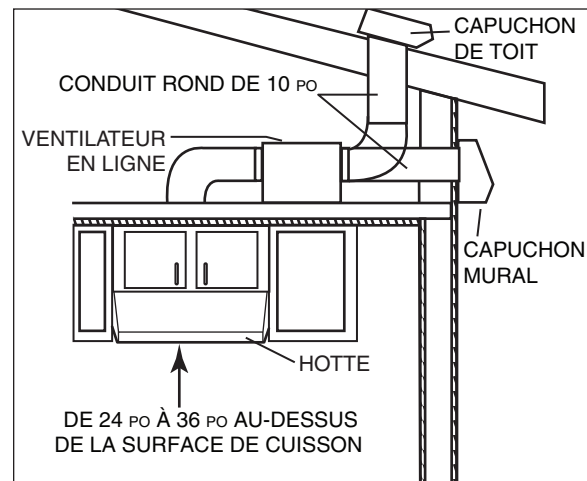
INSTALLATION TYPE VENTILATEUR EN LIGNE MODÈLE ILB6, ILB9 OU ILB11
