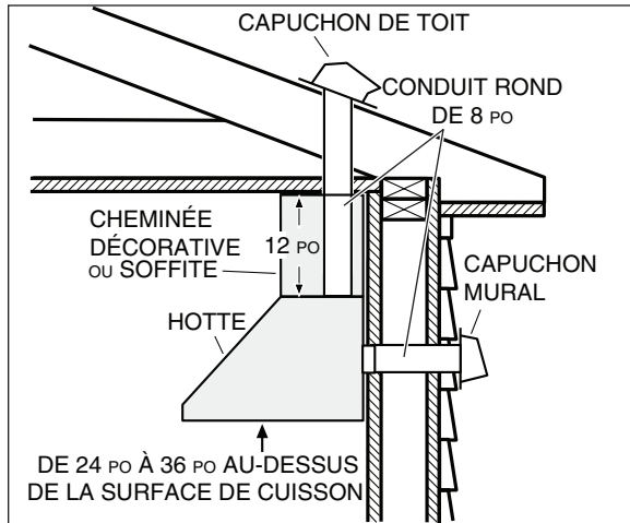
INSTALLATION TYPE VENTILATEUR INTÉRIEUR SIMPLE MODÈLE iQ6
