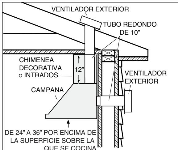
INSTALACIÓN HABITUAL CON EL VENTILADOR EXTERIOR EB9 O EB15
