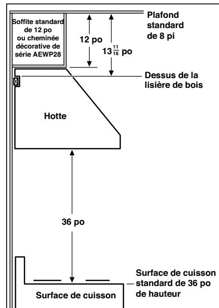
INSTALLATION AVEC UN SOFFITE STANDARD DE 12 PO OU UNE CHEMINÉE DÉCORATIVE OPTIONNELLE DE SÉRIE AEWP28
