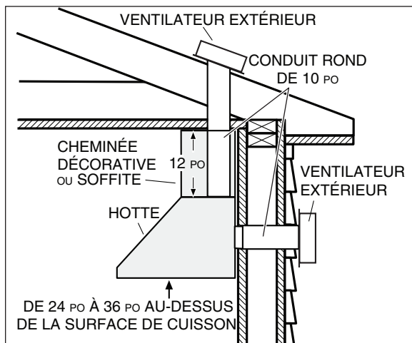
INSTALLATION TYPE VENTILATEUR EXTÉRIEUR MODÈLE EB9 OU EB15
